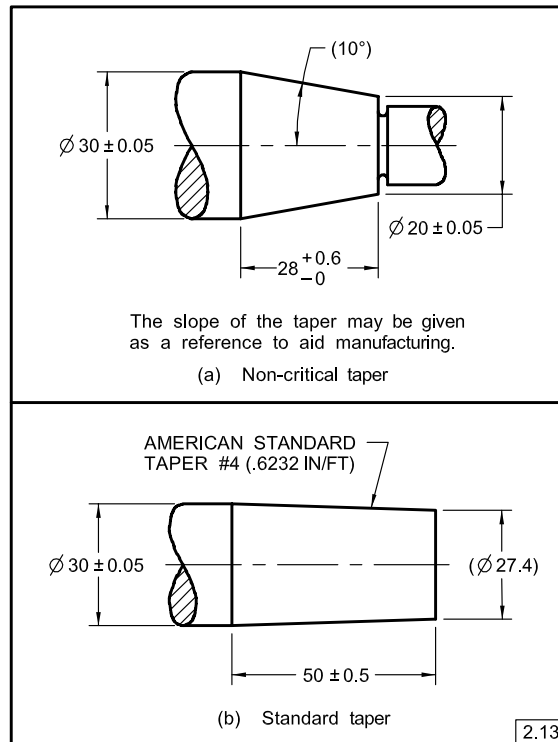
Fig. 2-19 Specifying Tapers
